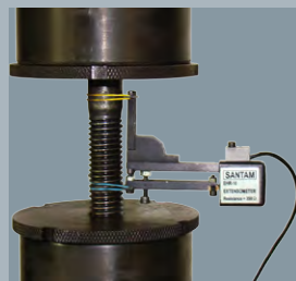
Stud Bolt
