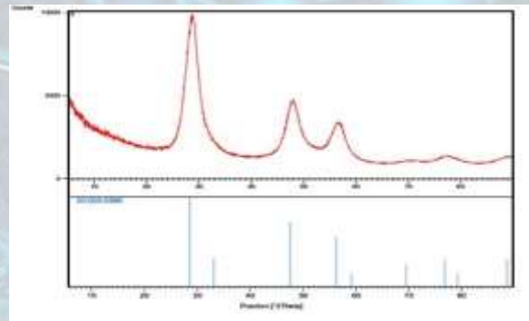
طیف پراش پرتو ایکس
