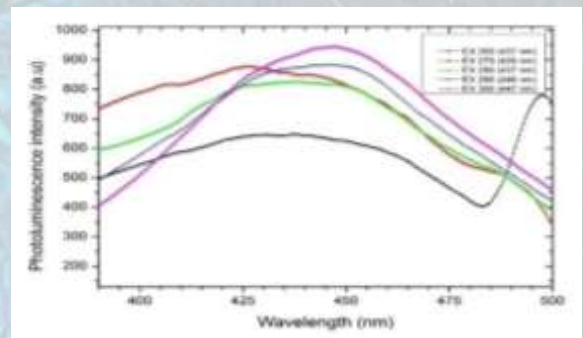
طیف PL در طول موج ۴۰۰-۵۰۰ nm
