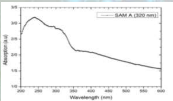
طیف جذب در طول موج ۲۰۰-۶۰۰ nm
