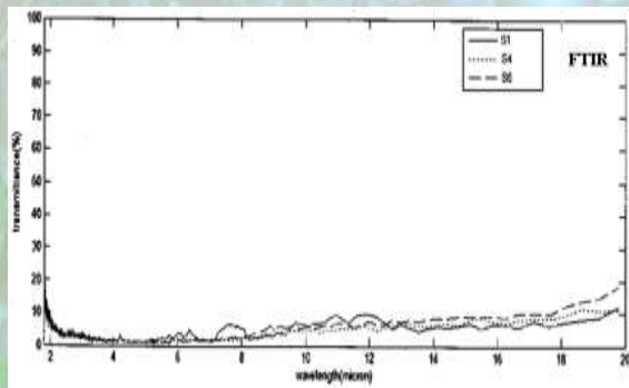
طیف FTIR
