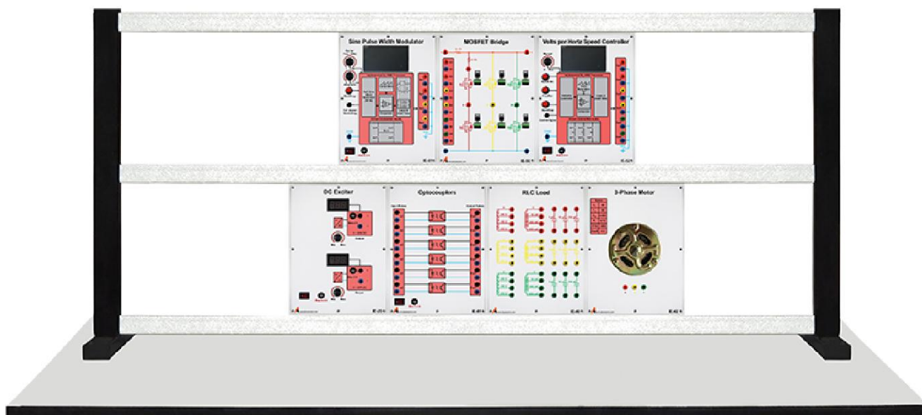
آموزنده الکترونیک صنعتی اینورتر و کنترل (V/f (106-IE
