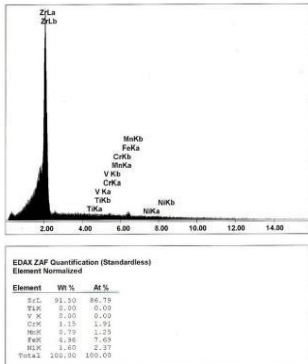
نمودار EDX زیرکونیا
