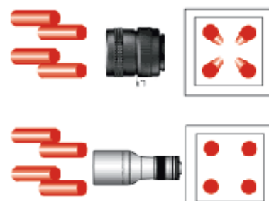
تصویر دریافتی از لنز معمولی و لنز Telecentric
