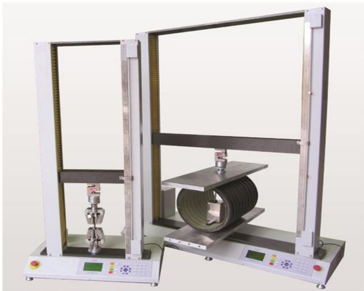
دستگاه تست کشش یونیورسال مدل SBN-20KN سیستم سرو الکتریکال
