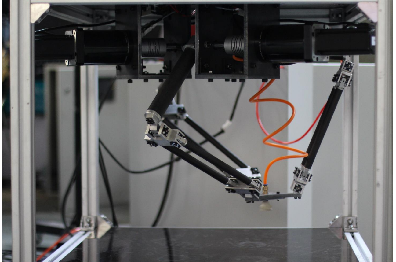
مجموعه ربات دلتا سه درجه آزادی
