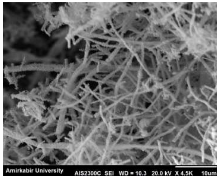
نانوالیاف سرامیکی
