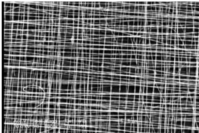
نانوالیاف بافت ۹۰ درجه (توسط جمع کننده سفارشی)
