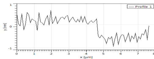
آنالیز AFM گرافن اکسید سنتز شده
