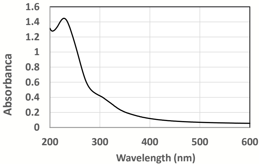
طیف UV-Vis گرافن اکسید سنتز شده
