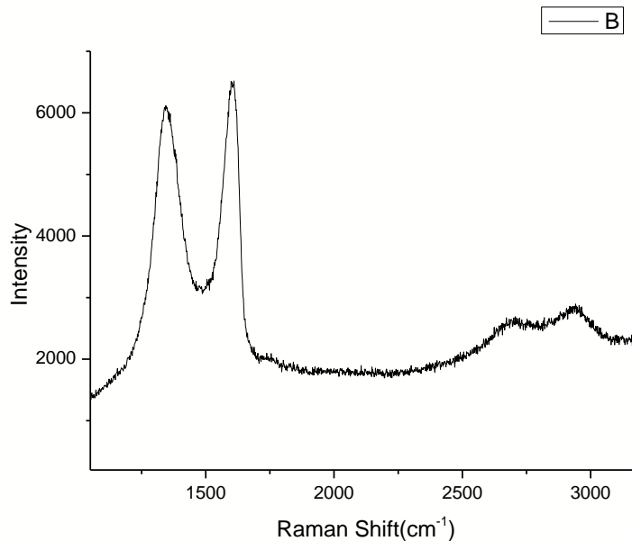
آنالیز رامان اسپکتروسکوپی گرافن اکسید سنتز شده
