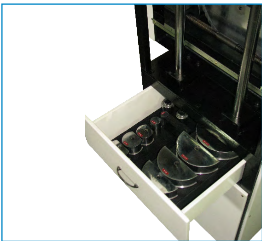
آداپتورهای فک خمشی با قطرهای مختلف
