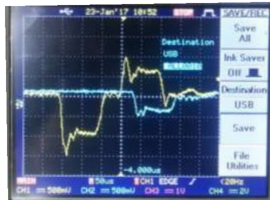
نمایی از موج های Transmitted, Reflected, Incident
