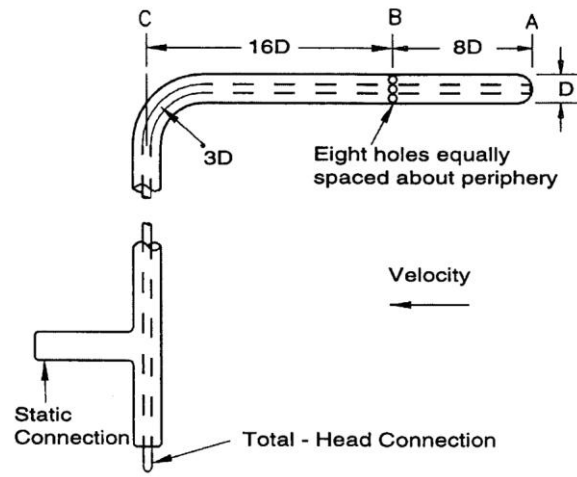
لوله پیتوت استاندارد
