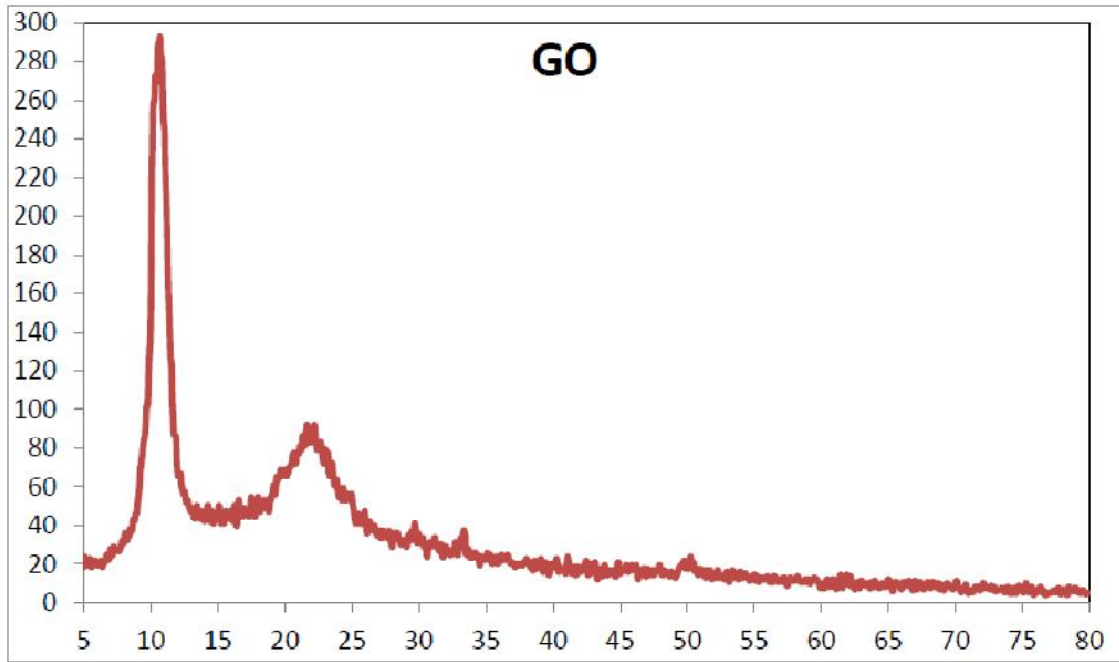
طيف XRD
