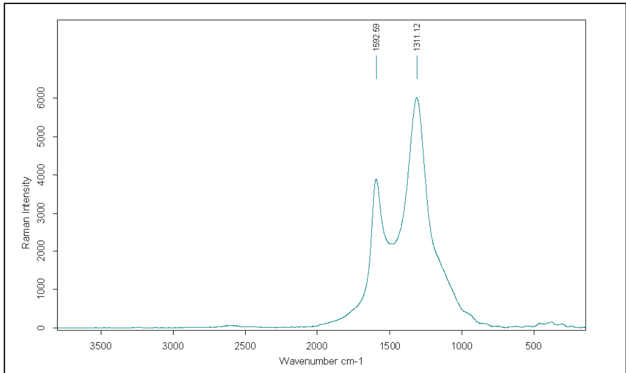
طيف رامان
