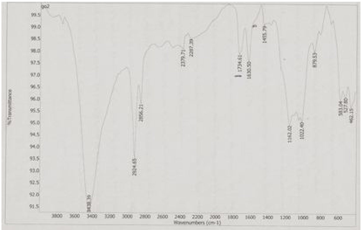
طيف IR
