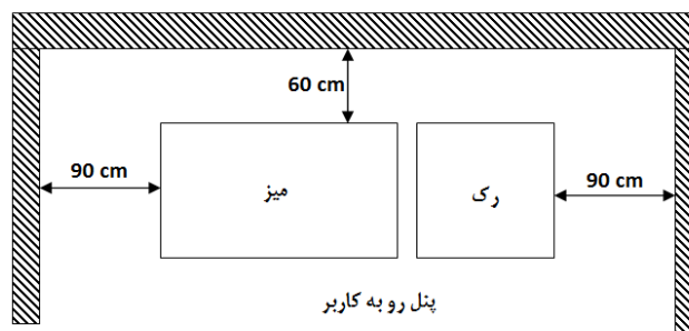
شکل (۱). فاصله مورد نیاز سامانه از دیوار
