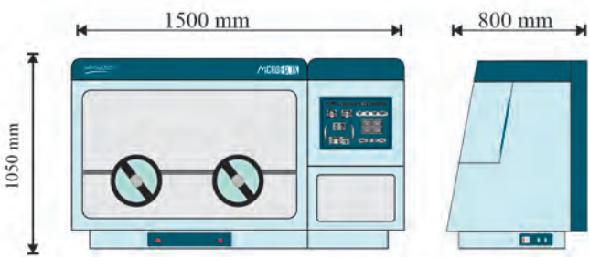
ابعاد مرسوم
