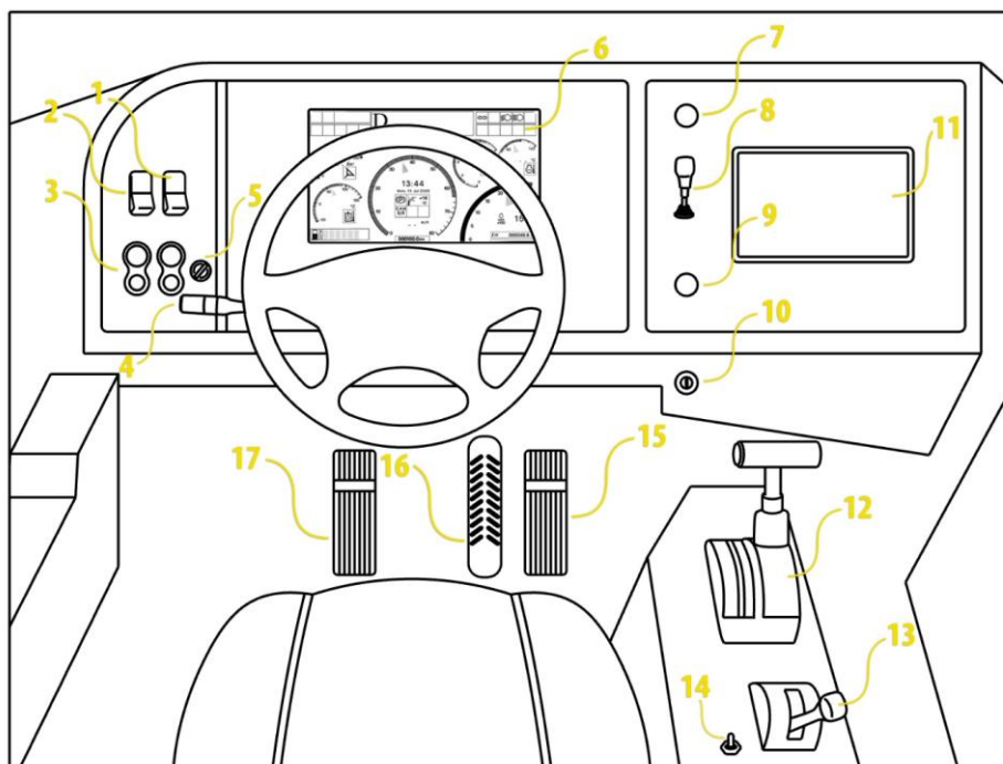
شکل ۳- ادوات داخل کابین شبیه‌ساز رانندگی دامپ‌تراک (ساخت ایران - شرکت فناوری شبیه‌ساز نصیر)
