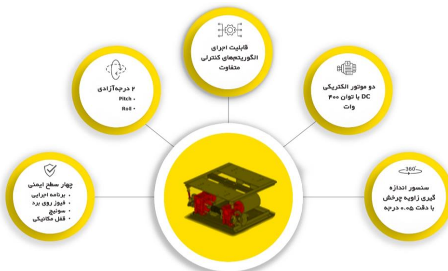
شکل ۱۳- قابلیت‌ها و مشخصات سیستم حرکتی دو درجه آزادی صندلی
