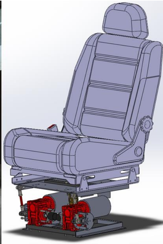
شکل ۱۴- پیاده‌سازی سیستم حرکتی دو درجه آزادی برای صندلی اپراتور به صورت بومی (ساخت ایران - شرکت فناوری شبیه‌ساز نصیر)
