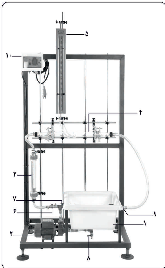
اجزاء دستگاہ اوریفیس متر
