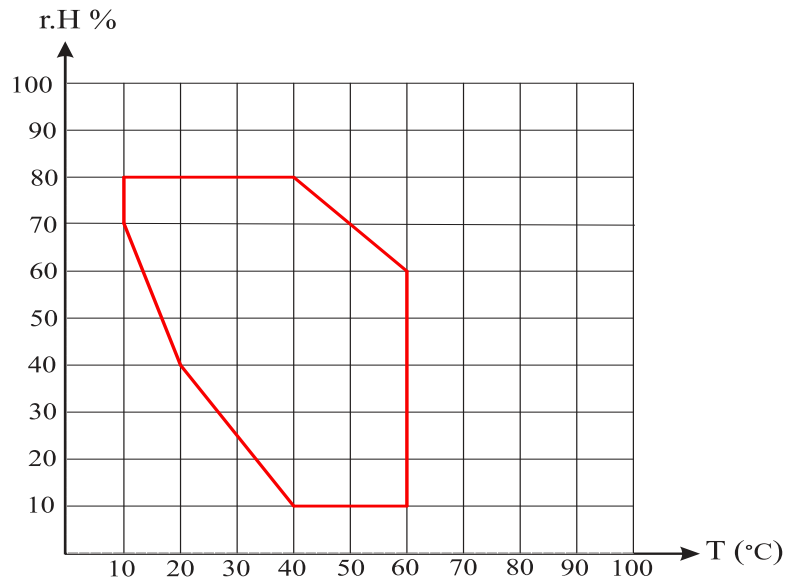
نمودار دما و رطوبت بدون کاست نوری
