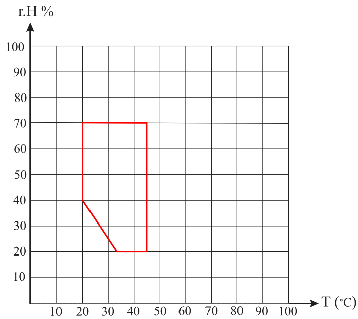
نمودار دما و رطوبت با لامپ روشن
