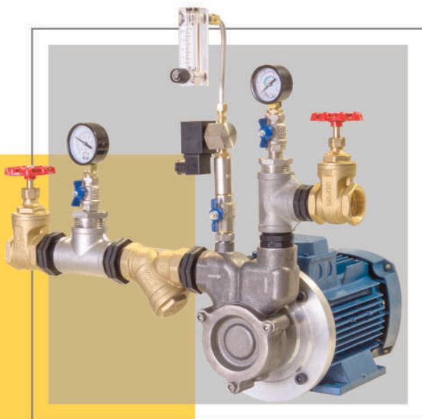
پمپ ورتکس دوفازی نانو حباب ساز (آزمایشگاهی)
