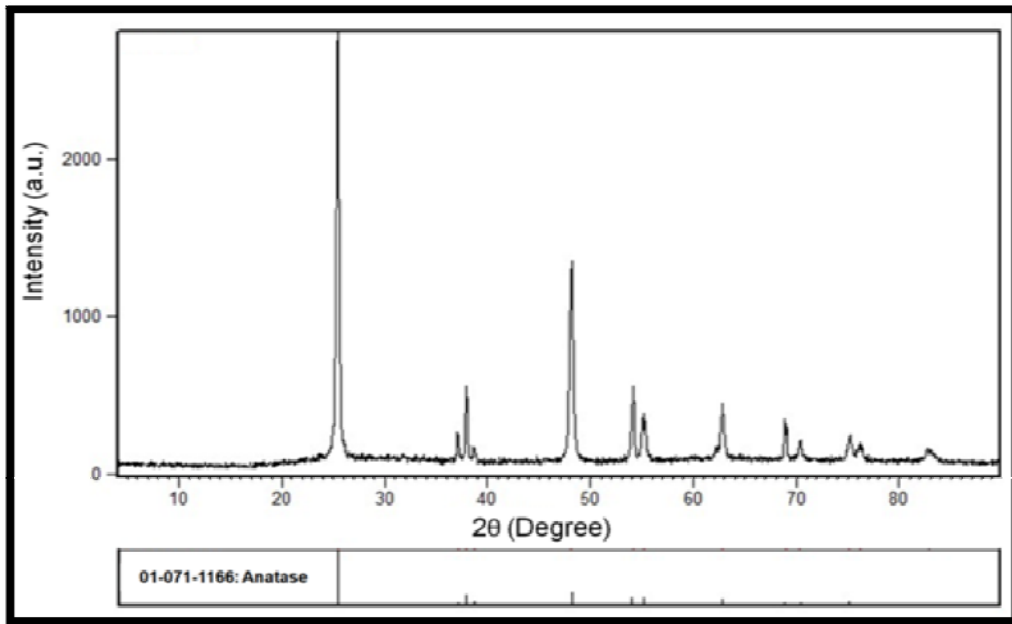
تصویر XRD
