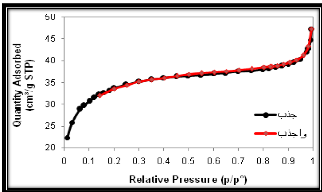
BET
