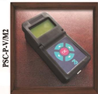
سامانه تست و کالیبراسیون حسگر مقاومتی گاز قابل حمل
