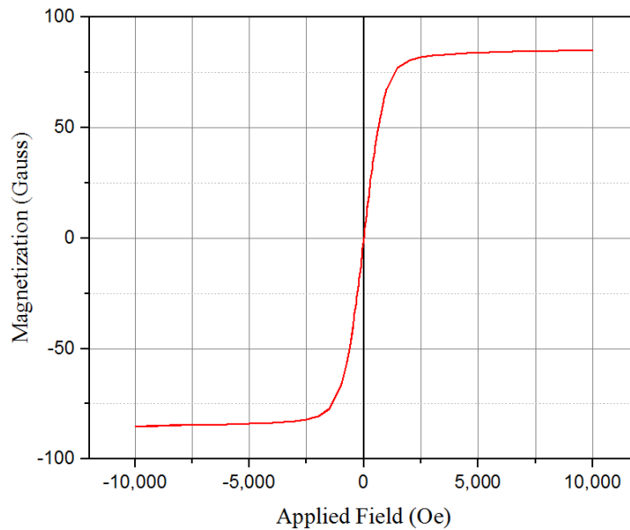
مغناطش اشباع بر حسب میدان مغناطیسی.
