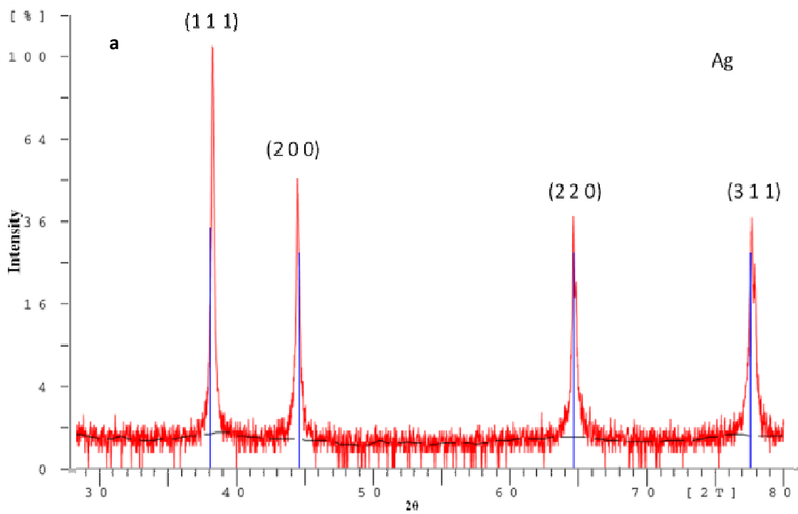
آنالیز XRD نانوپودر نقره
