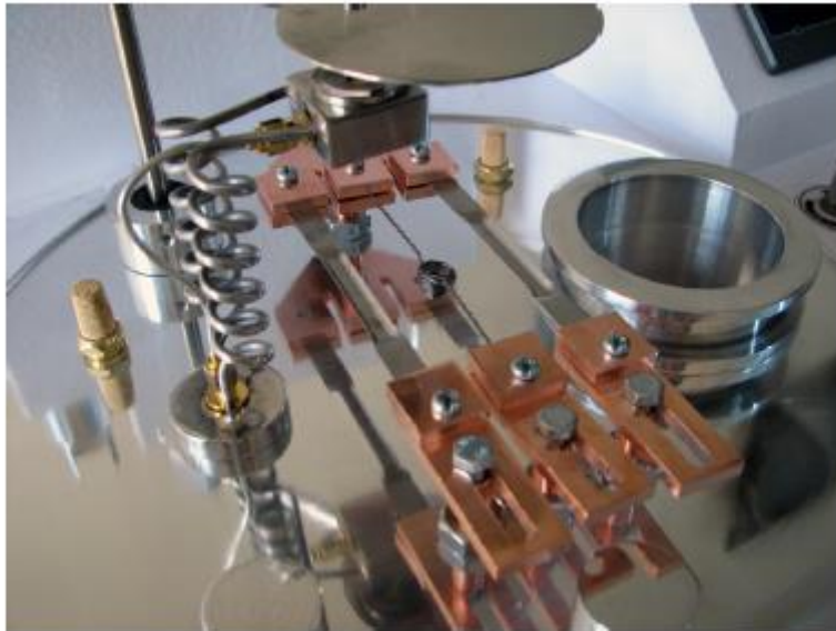
نمایی از داخل محفظه تبخیر حرارتی
